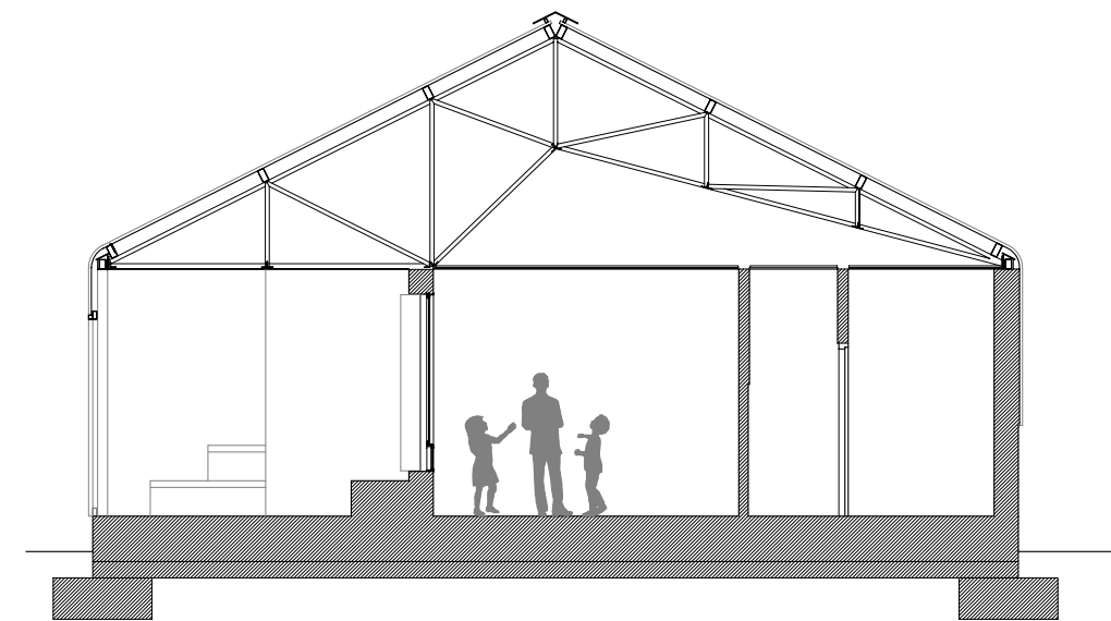
sección transversal
