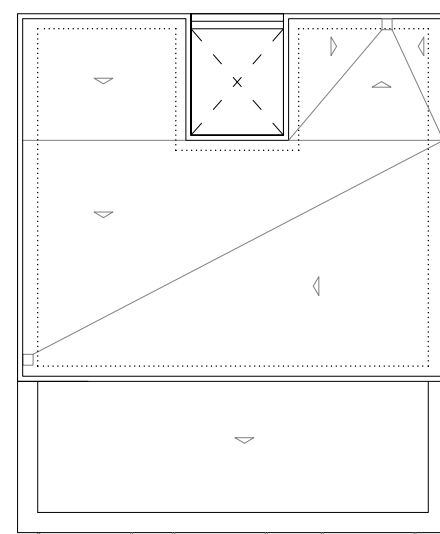
planta cubierta
