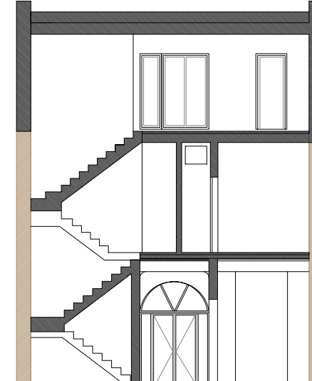
sección
