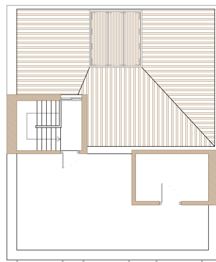
planta ático
